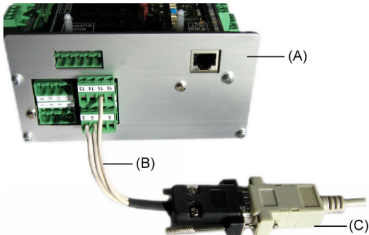
Steuerung (A), Flash-Kabel (B), Nullmodemkabel (C)
