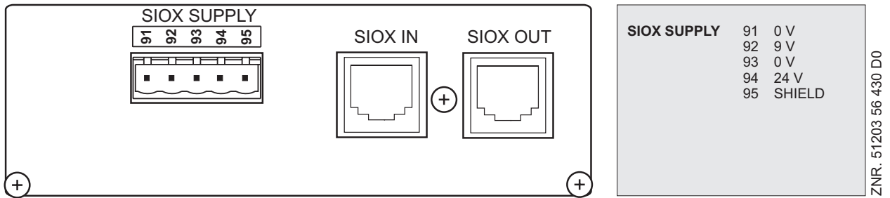
Klemmenbelegung SIOX-Erweiterungsmodul - Anschlüsse seitlich
