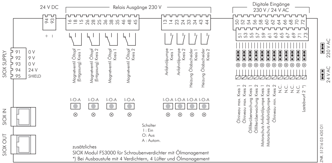
Klemmenbelegung für zusätzliches SIOX-Erweiterungsmodul (wird für Ölmanagement verwendet)
