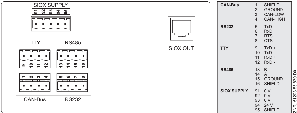
Klemmenbelegung Grundmodul FS 3000 - Anschlüsse seitlich
