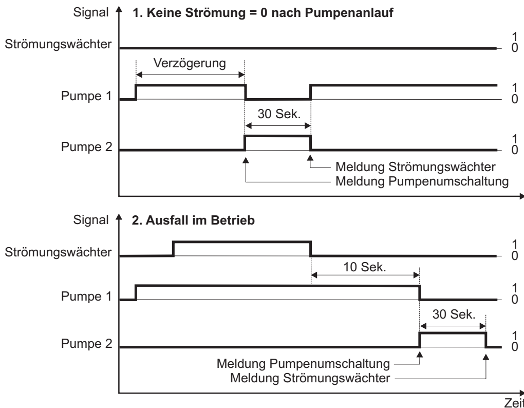
FS 3000 Strömungswächter
