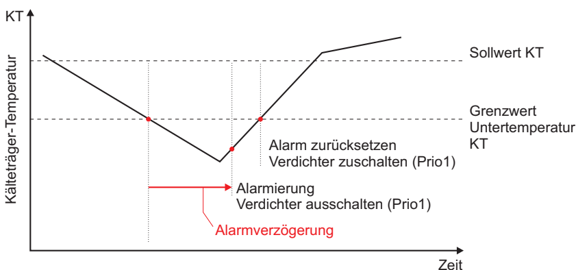
FS 3000 Überwachung Kälte-träger-Temperatur (KT)
