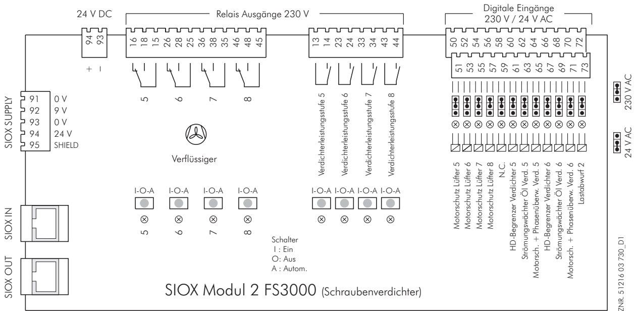
Klemmenbelegung 2. SIOX-Modul: Ein-/Ausgangs-Erweiterung für Schraubenverdichter
