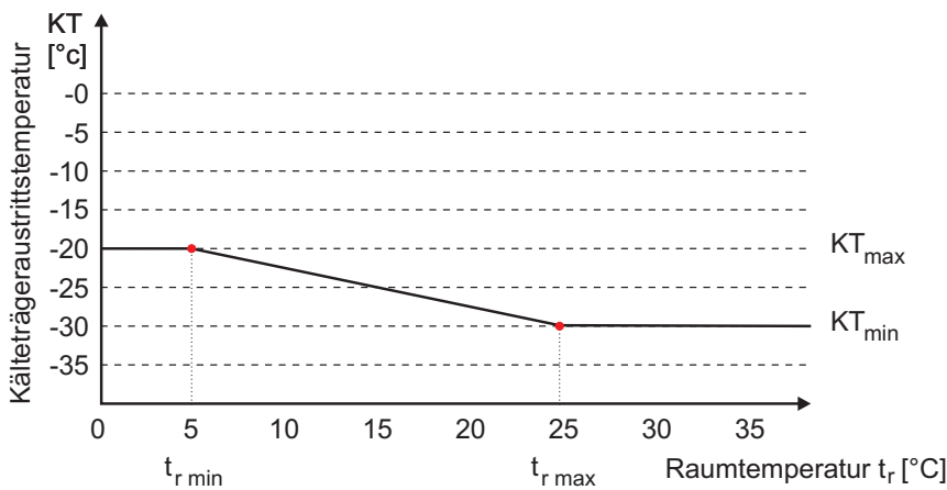
Regelung Kälte­trä­ger­aus­tritt­tem­pe­ra­tur Sollwertberechnung
