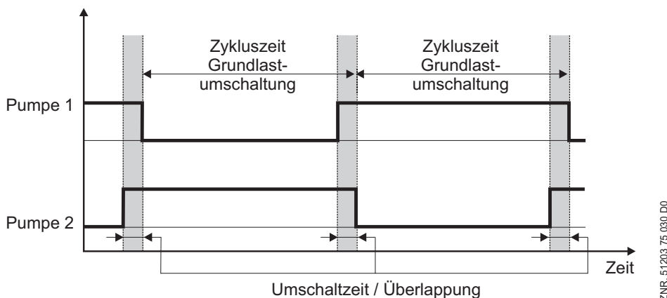
FS 3000 Pumpenumschaltung
