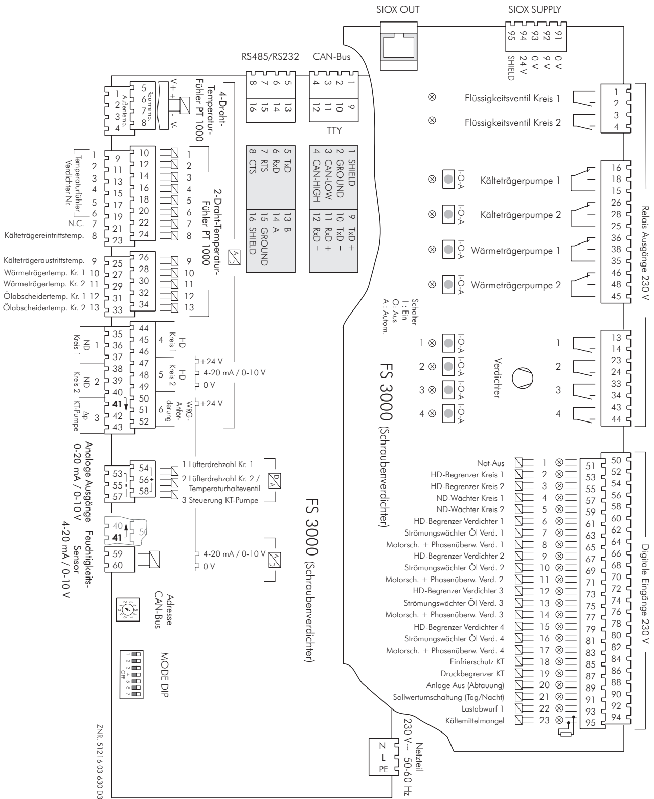
Klemmenbelegung Grundmodul FS 3000 für Schraubenverdichter
