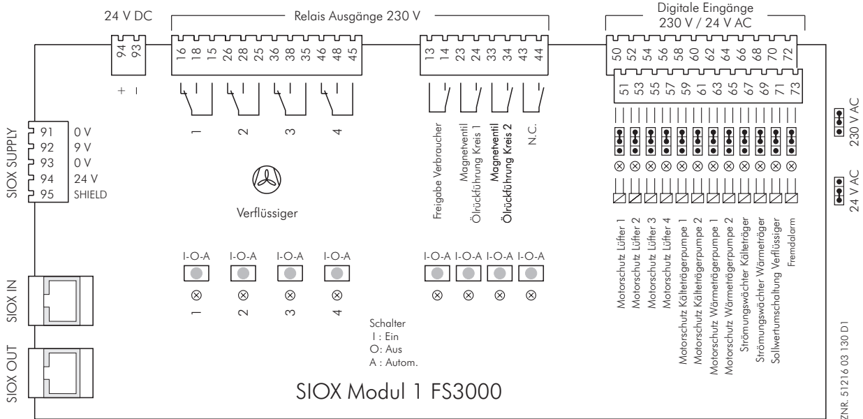
Klemmenbelegung 1.SIOX-Modul: Grundausbau FS 3000
