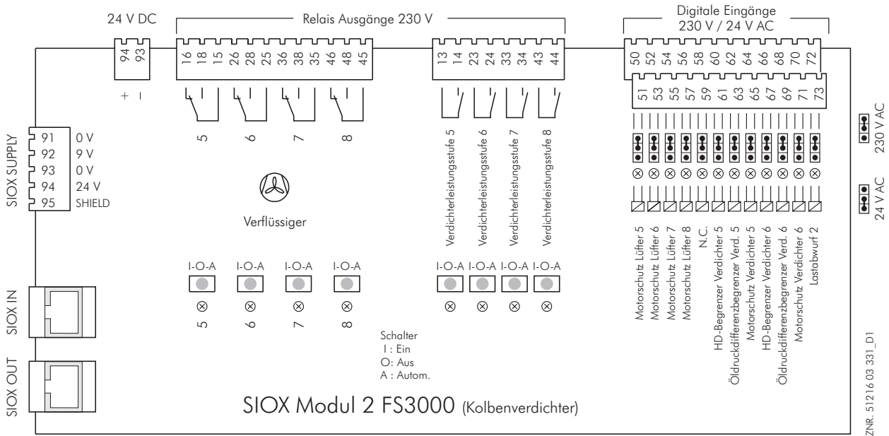
Klemmenbelegung 2. SIOX-Modul: Ein-/Ausgangs-Erweiterung für Kolbenverdichter
