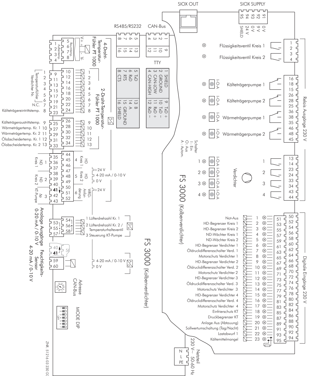
Klemmenbelegung Grundmodul FS 3000 für Kolbenverdichter
