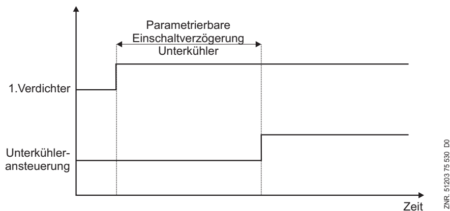
FS 3000 Unterkühlersteuerung
