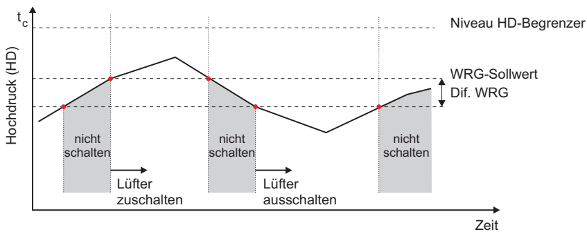
FS 3000 Regelalgorithmus WRG-Betrieb Wärmeträgerregelung
