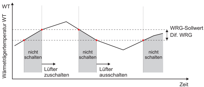
FS 3000 Regelalgorithmus WRG-Betrieb Wärmeträgerregelung
